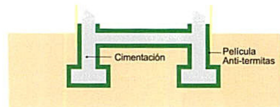
2 La barrera se acopla perfectamente a la cimentación imposibilitando el ataque de termitas
