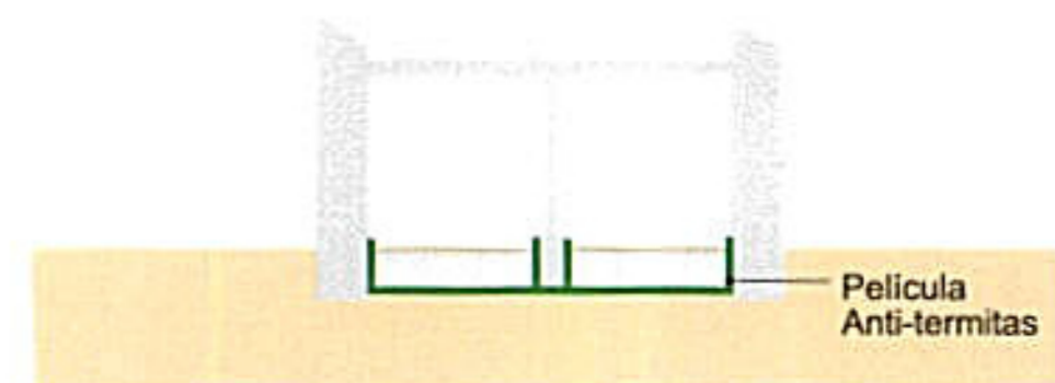
1 Se levanta el suelo del edificio y antes del relleno y el hormigón se coloca la barrera, aislando perfectamente el edificio de la tierra
