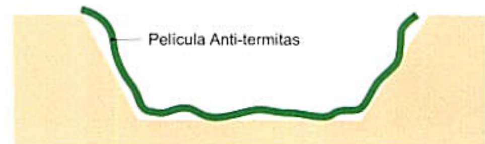
1 Antes de la cimentación se cubre toda la superficie con TERMIFILM
