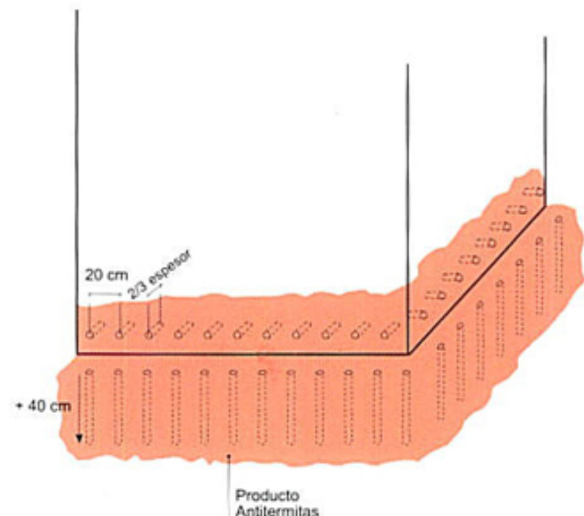
Barrera antitermitas
